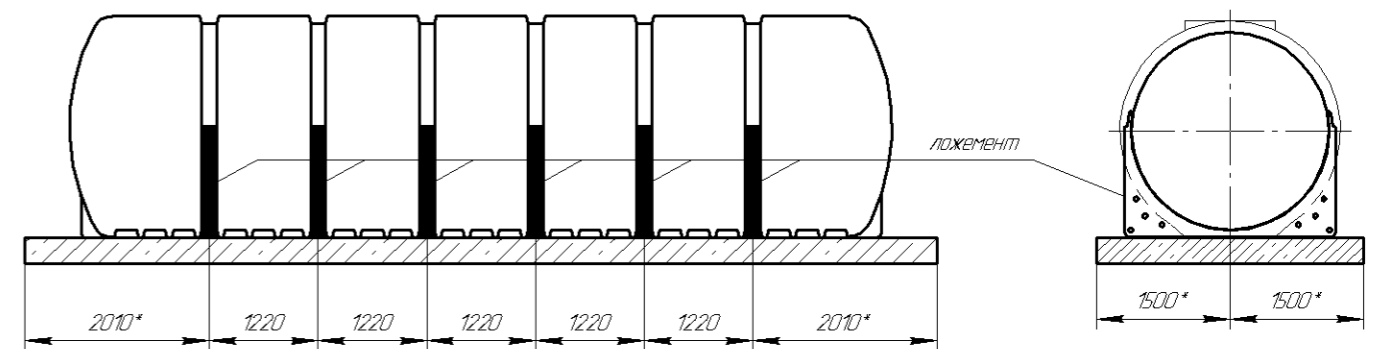
Схема установки ложементов
